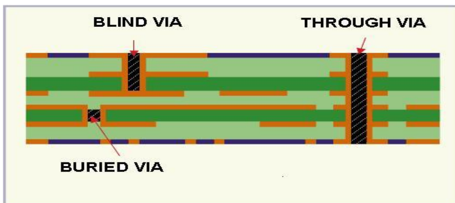
Obr. 3: Druhy propojovacích technologií vícevrstvých spojů. [14]
