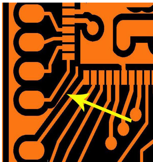
Obr. 8: Zbytečné rozlití mědi v blízkosti spoje.[8]
