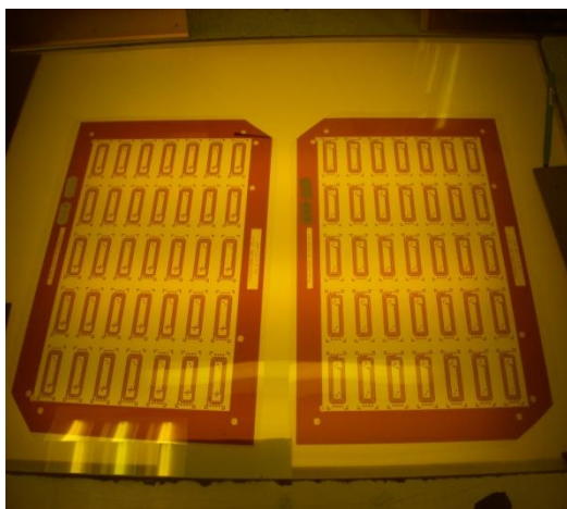
Obr. 32: Diazo filmy.
